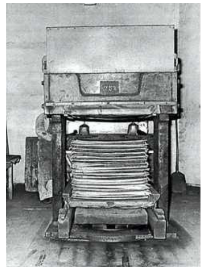
Schwarzpulver-Stapelpresse in der Pulverfabrik Kunigunde; Foto: WANO GmbH Kunigunde
